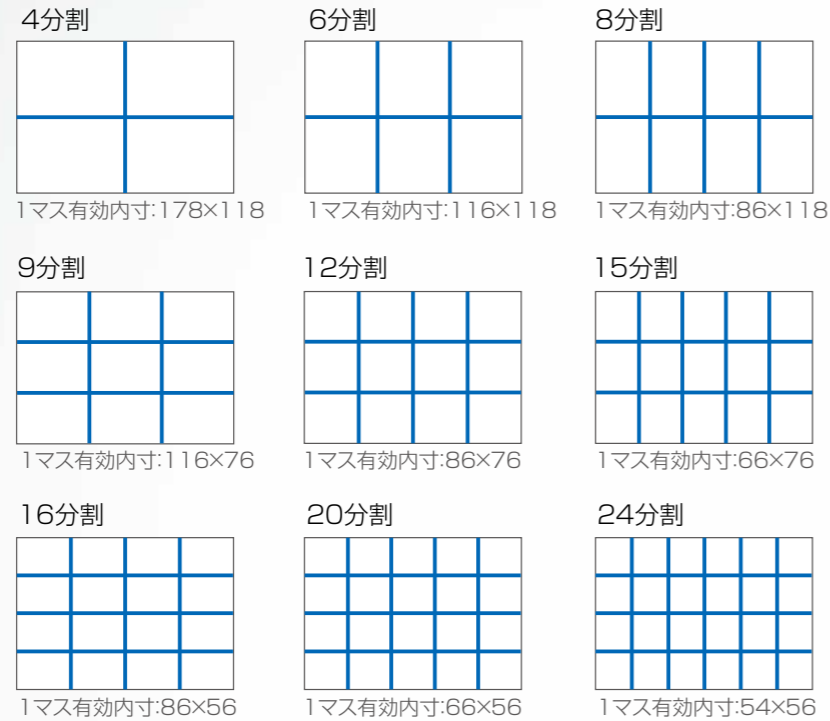
TC-1の仕切りパターン(例)
