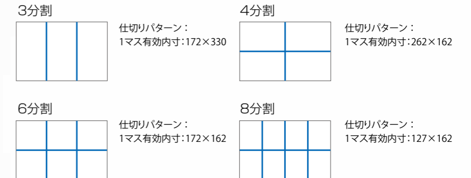
TR-22、TR-27、TR-37、TR-47の 仕切りパターン(例)
